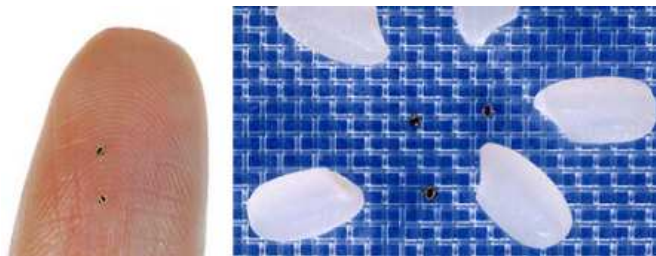
(Der RFID-Chip von Hitachi (2006) zur Kennzeichnung von Produkten, Tieren und Menschen ist nur 0.4 x 0.4 mm groß und hat selbst die Antenne integriert Größenvergleich: linker Bildteil: Chip auf Finger; rechter Bildteil: weiße Reiskörner zum Größenvergleich 10 )
